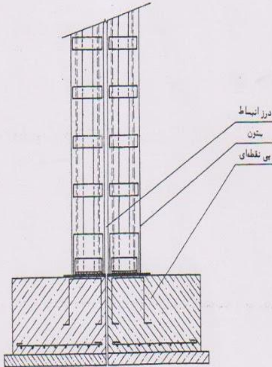
زوشن درمحل ستون و پی نقطه‌ای
